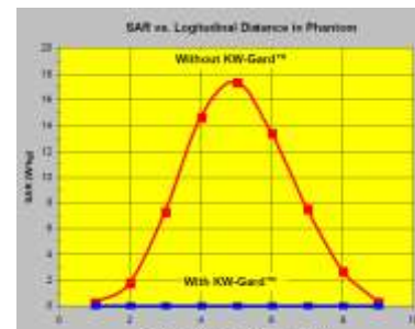
ファントムからの距離と SAR 赤: 未着用時 青: 着用時
