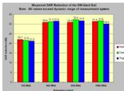
着用時の SAR 低減効果 赤: 頭部、緑: 胸部、青: 大腿部
