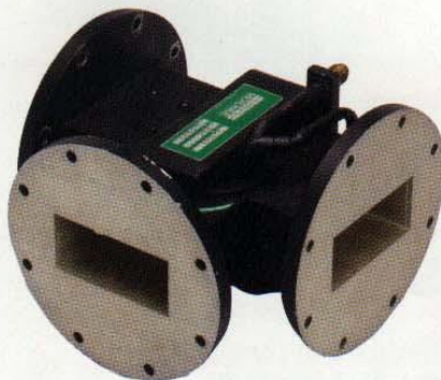
WR 284
