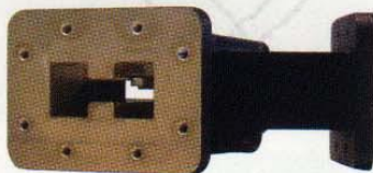
WRD 350 4 – 8GHz
